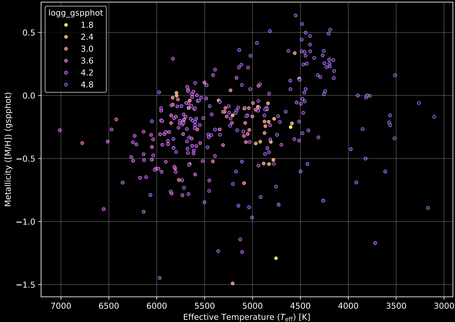
APOGEE DR17 Field: [N4147] Stellar Population Parameters (n= 307)
